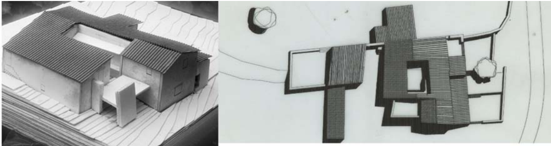
Maqueta i planta coberta de la proposta de consolidació selectiva dels volums originals.
